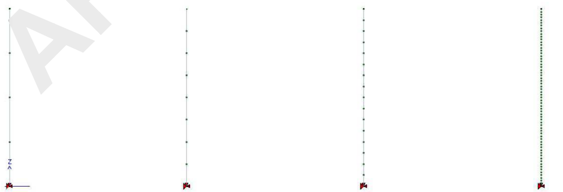
Figura 6: Modelli FEM: A, B, C, D (da sinistra a destra)
