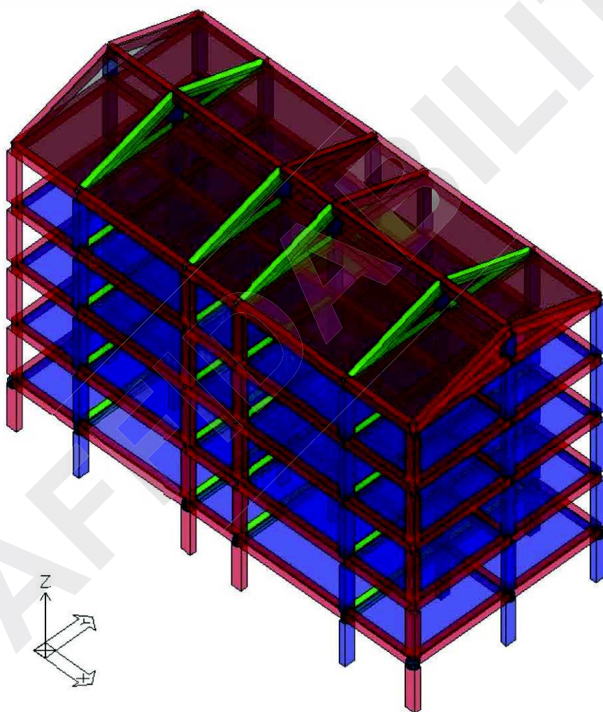
STRUTTURA TRIDIMENSIONALE UTILIZZATA PER LA VALIDAZIONE
