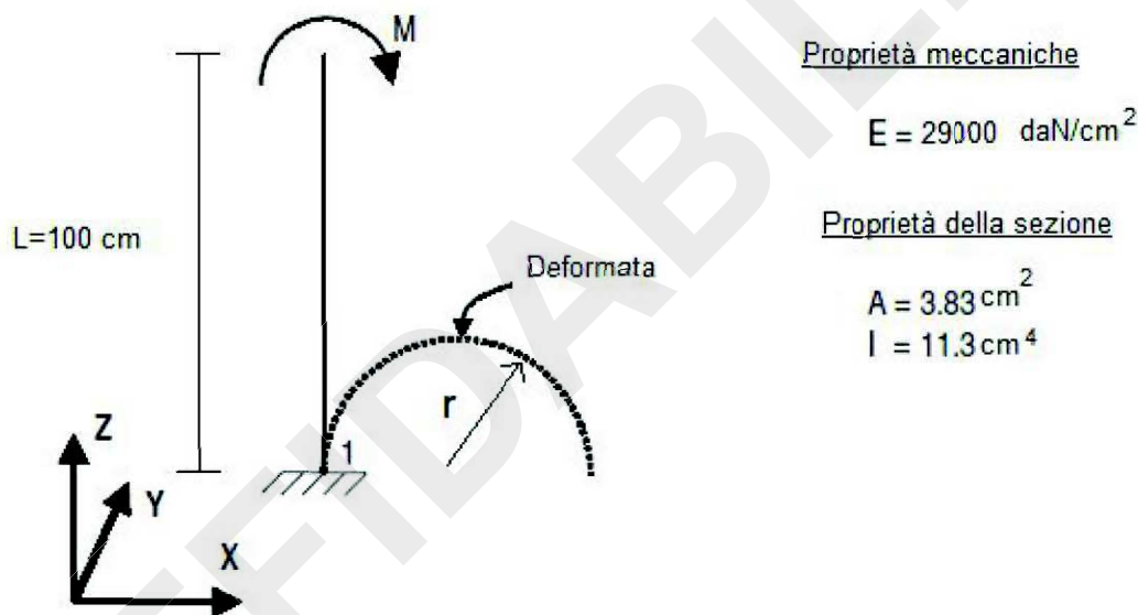
Figura 5: Schema statico
