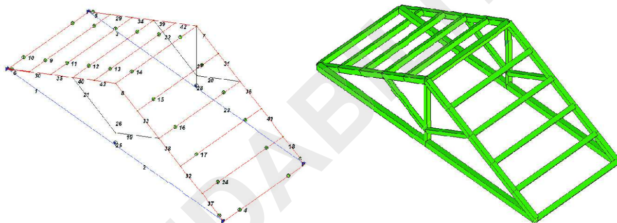
Figura 1 – Copertura in legno: vista filo di ferro e solido accurato
