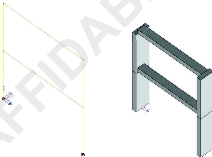
Figura 1 – portale a due piani in c.a.: vista filo di ferro e vista solida
